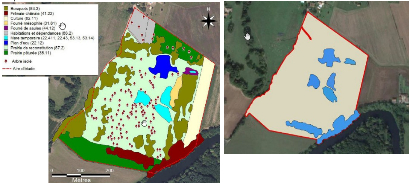
Cartographie des habitats à gauche (source : étude d'impact, p. 61) : Carte de synthèse des zones humides à droite (source : étude d'impact, p 77)
