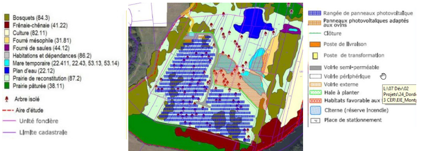
Superposition du projet avec les habitats naturels - extrait étude d'impact page 164
